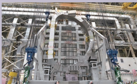
TFコイルが垂直に立ち上がる
