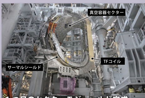
1つ目のセクターモジュールが完成
