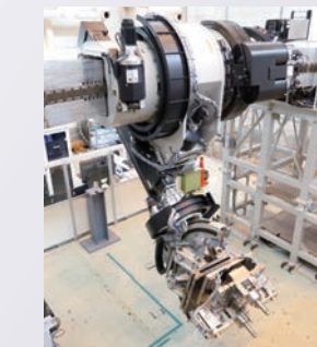
核融合炉保守点検用のロボットアーム
