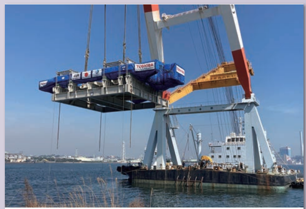
TF コイル 8 機目の出荷の様子
